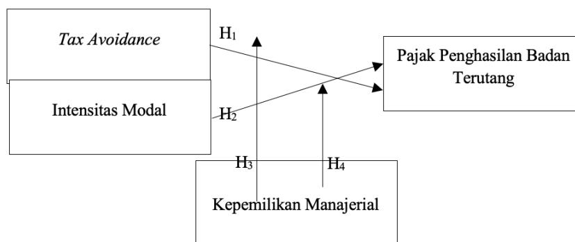
Gambar 2. Kerangka Konseptual
